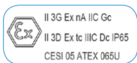
Etichetta marcatura ATEX
