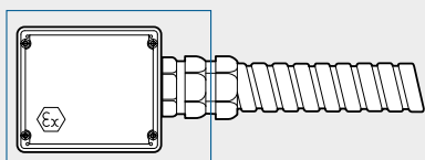
Cassetta di derivazione CT + raccordo pressacavo SILOK ATEX
